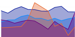
Superposición
